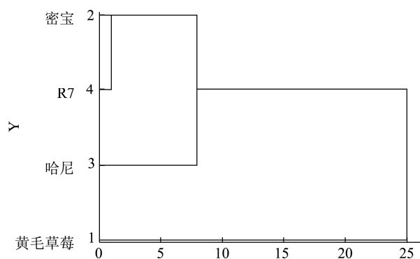
图3 4种草莓香气主成分聚类分析
