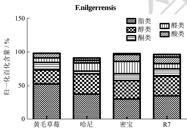
图 2 4 种草莓品种香气成分分类比较
