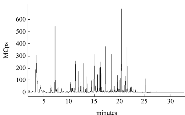
图 1 黄毛草莓挥发性物质 GC-MS 总离子流程图
