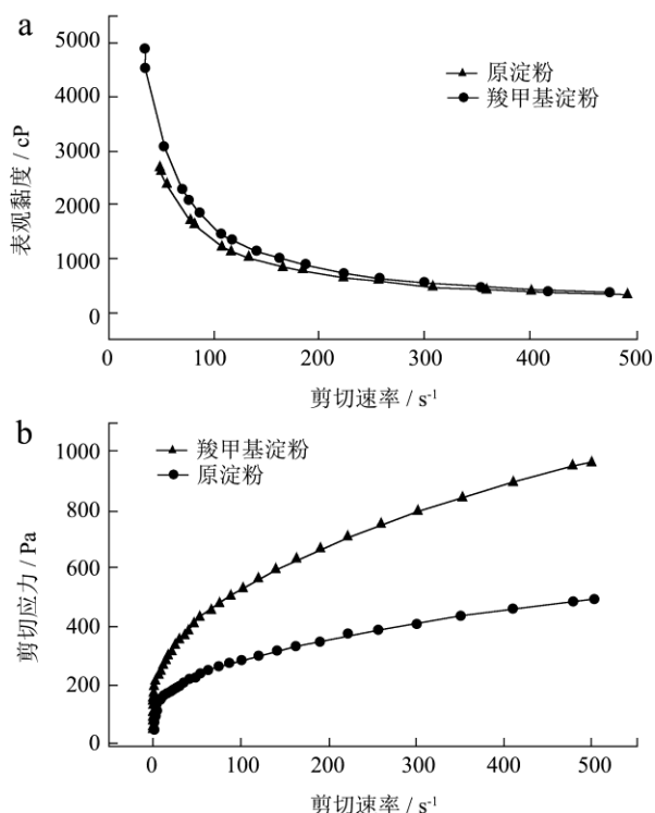
图 2 籼米淀粉和羧甲基籼米淀粉静态流变曲线
