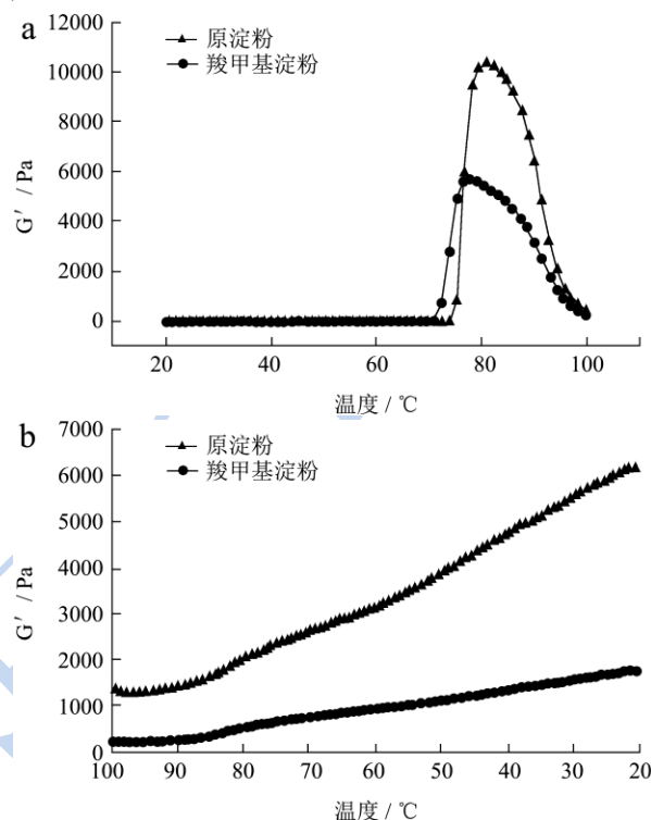
图 1 粳米淀粉和羧甲基粳米淀粉的 G' 随温度的变化曲线
