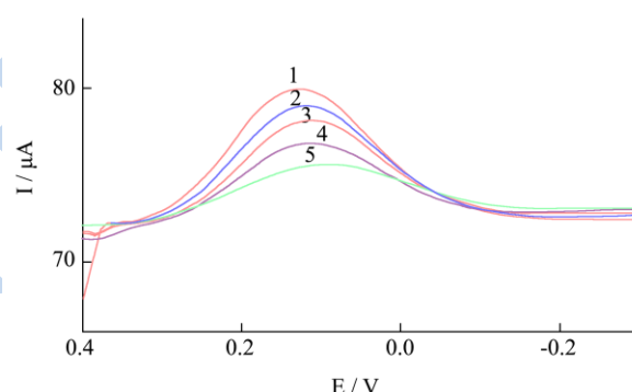
图 5 扫描次数对峰电流和峰电位影响
