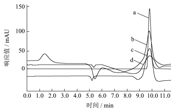
图 7 Acr 标品及 3 种油炸样品 HPLC 图
