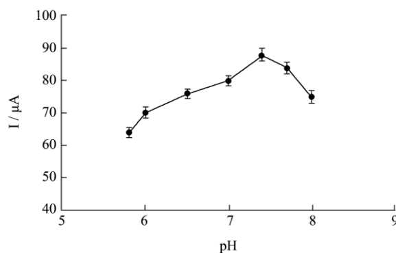
图 4 支持电解质 pH 对峰电流影响
