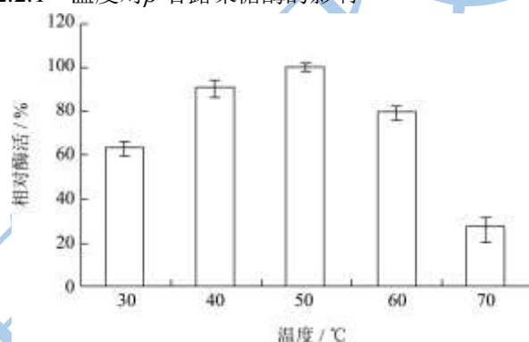
图8 不同反应温度对酶活的影响
