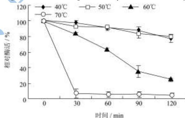
图9 不同反应温度对酶稳定性的影响
