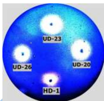
图7 UV-DES 诱变部分菌株的水解圈情况
