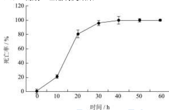
图3 硫酸二乙酯诱变时间死亡率曲线
