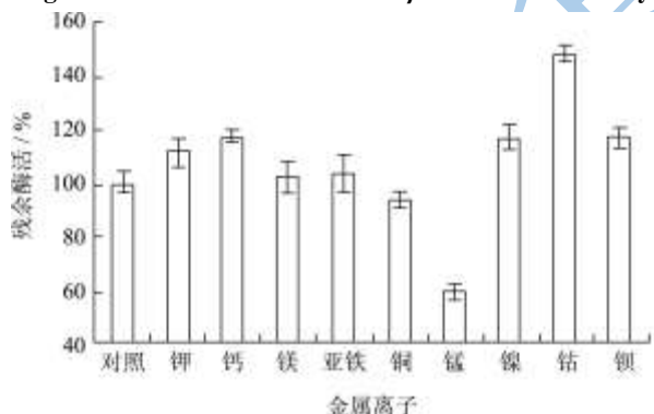
图 12 金属离子对酶稳定性的影响
