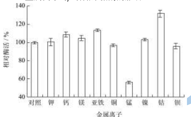
图 11 金属离子对酶活性的影响
