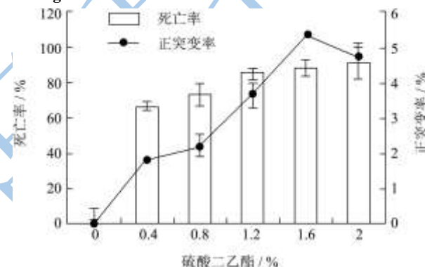
图4 不同DES剂量致死率和正突变率的曲线
