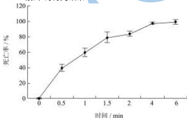
图2 紫外线诱变死亡率曲线
