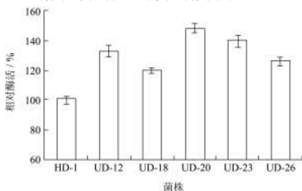
图6 图 DES-UV 复合诱变部分菌株酶活
