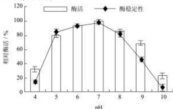
图 10 不同 pH 对 \beta -甘露聚糖酶酶活和酶稳定性的影响
