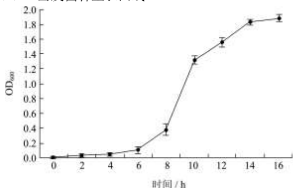
图1 菌体OD 600 随培养时间的变化
