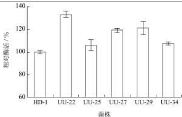
图5 紫外线-光复活诱变部分菌株酶活
