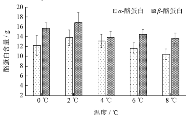
图 3 冷却温度对不同酪蛋白分离的影响
