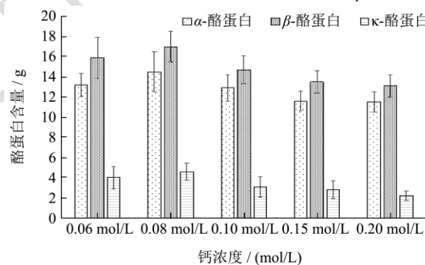
图2 不同钙离子浓度对不同酪蛋白分离的影响
