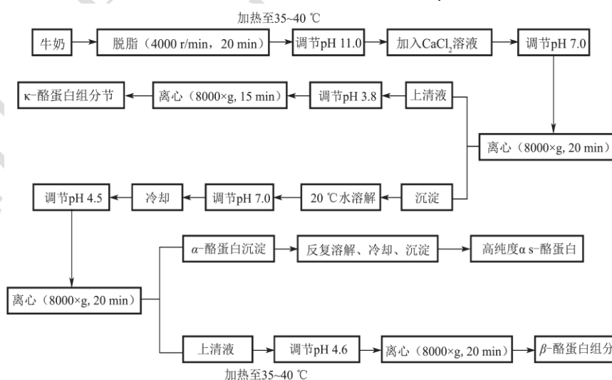
图1 \alpha -、 \beta -、 \kappa -酪蛋白分离工艺流程
