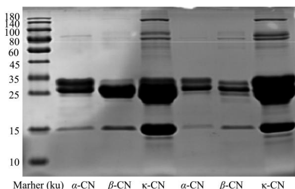
图 4 牦牛奶 α-、β-、κ-酪蛋白分离效果
