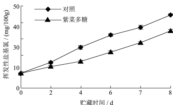
图 3 贮藏时间挥发性盐基氮变化
