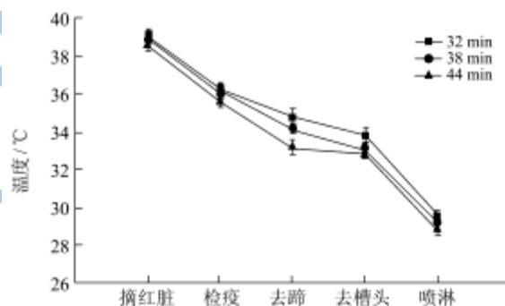
图 1 不同在轨时间条件对腔体内部温度的影响 (电击晕)
