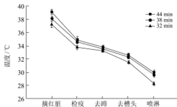
图 2 不同在轨时间对腔体内部温度的影响 (CO 2 致晕)
