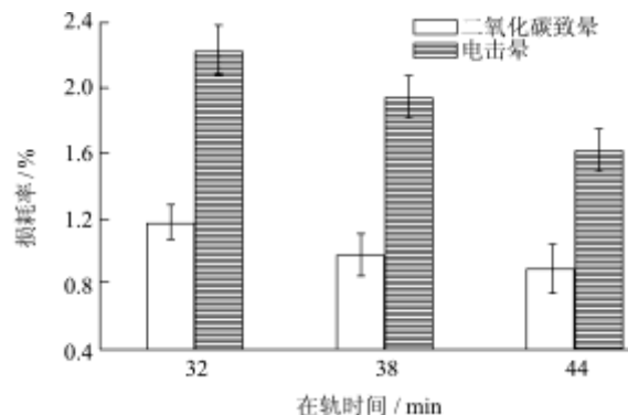
图3 不同在轨时间对预冷损耗的影响
