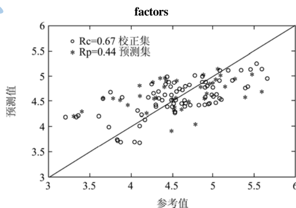
图 2 偏最小二乘回归模型预测结果
