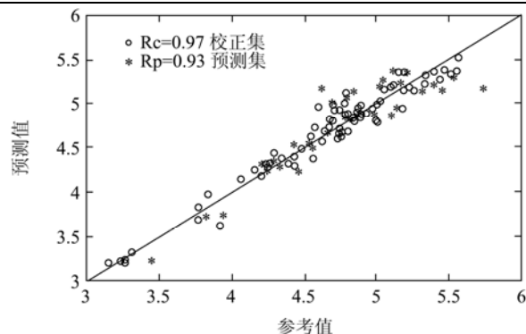
图4 BP神经网络模型预测结果
