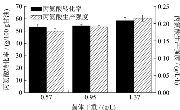
图 5 热诱导时机对 B0016-060BC 菌株 L-丙氨酸合成的作用
