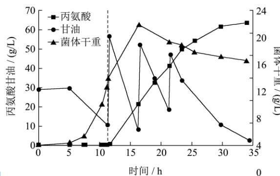
图 6 菌株 B0016-060BC L-丙氨酸发酵过程
