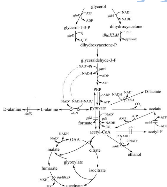
图 1 Escherichia coli B0016-060BC 重组菌株发酵甘油产 L-丙氨酸过程中的主要代谢反应
