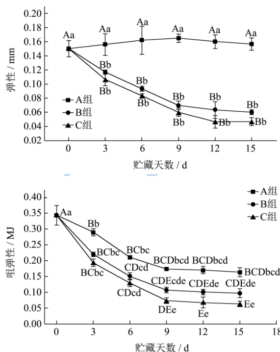
图 6 不同保鲜处理方法对于鱿鱼鱼肉弹性和咀嚼性的影响
