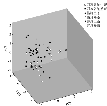
图 1 第 1、2、3 主成分得分图
