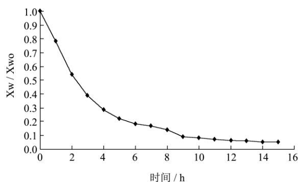
图2 牡蛎干燥过程中含水量的变化率
