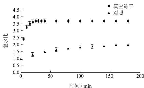
图3 冷冻干燥对牡蛎复水比的影响
