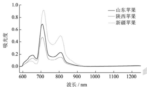
图2 不同地区苹果的近红外透射光谱
